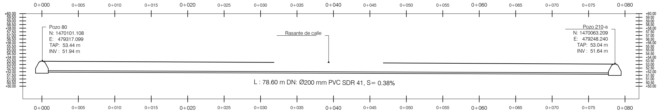
Perfil Red de Alcantarillado
