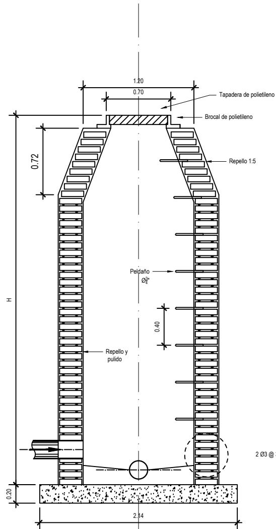
Pozo H: 3.51 a 4.10 m
