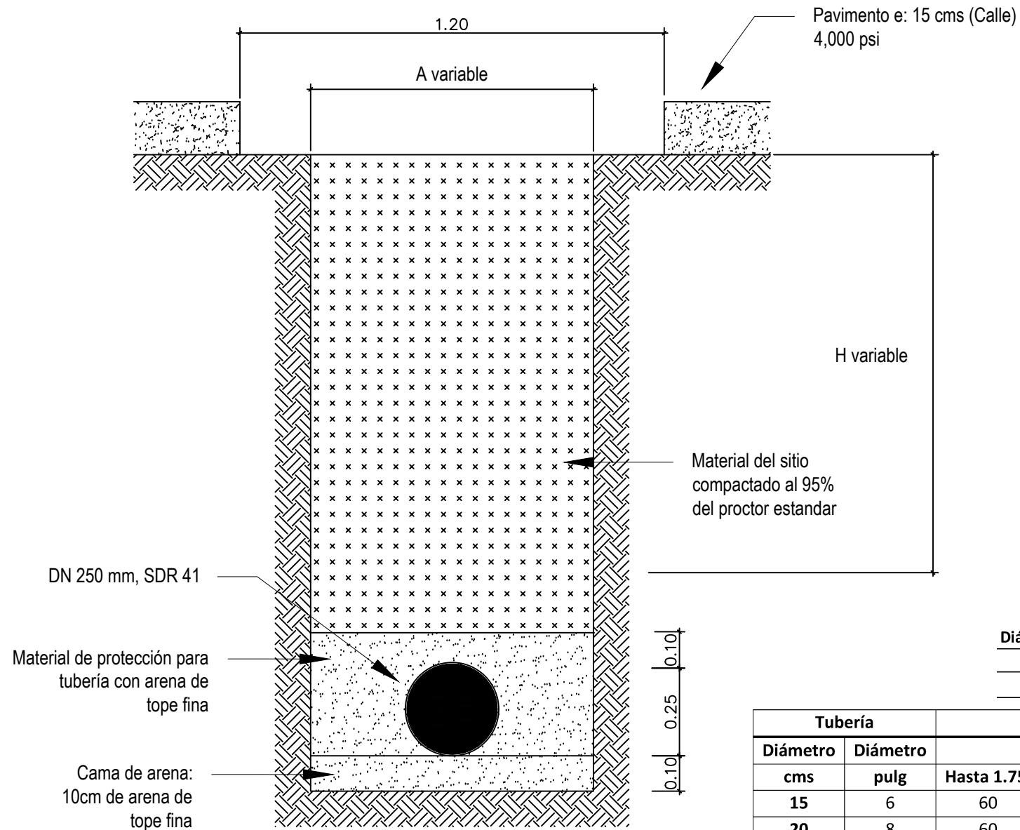
Zanja para tubería de red central
