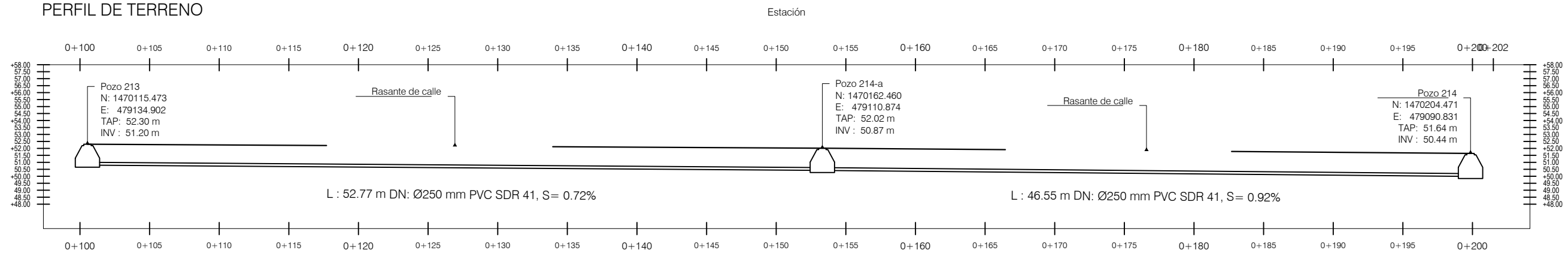
Perfil Red de Alcantarillado
